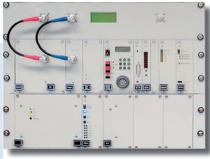
Ortsfeste Funkstelle FSO 416 (BOS 2m Band)
